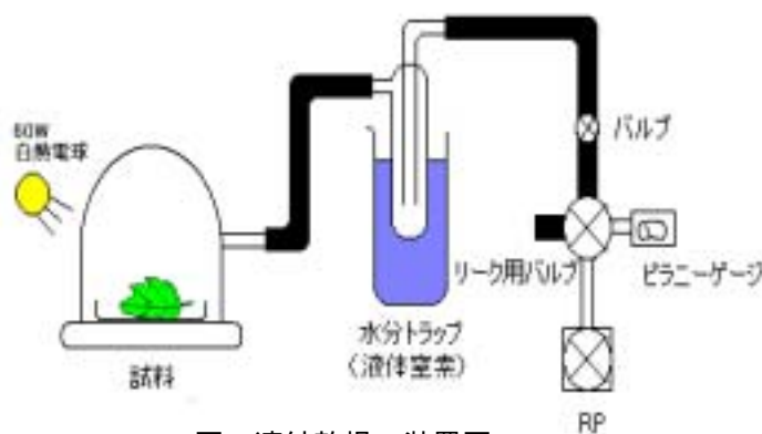
図 凍結乾燥の装置図
